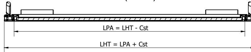
B-B ( 1:15 )
