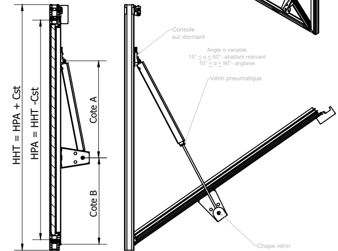
A-A ( 1:15 )
